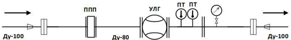
Рисунок 1 –Схема УУГ DN80 PN 6,3 МПа УУГ-Б-1-80-6,3-1/80
