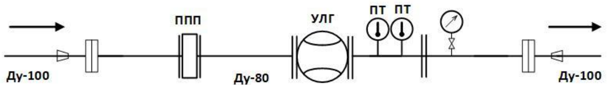
Рисунок 1 –Схема УУГ DN80 PN 10,0 МПа УУГ-Б-1-80-10,0-1/80
