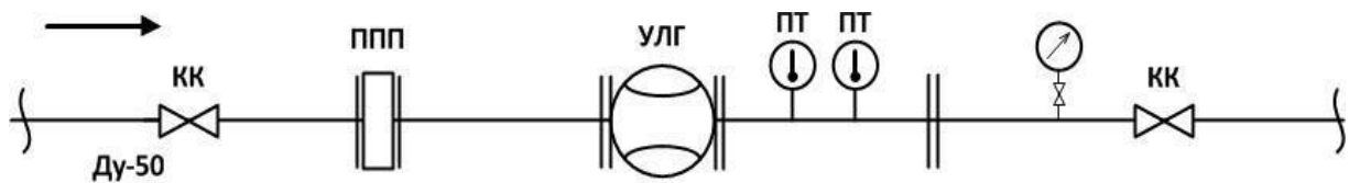
Рисунок 1 –Схема УУГ DN50 PN 6,3 МПа УУГ-Б-1-50-6,3-1/50
