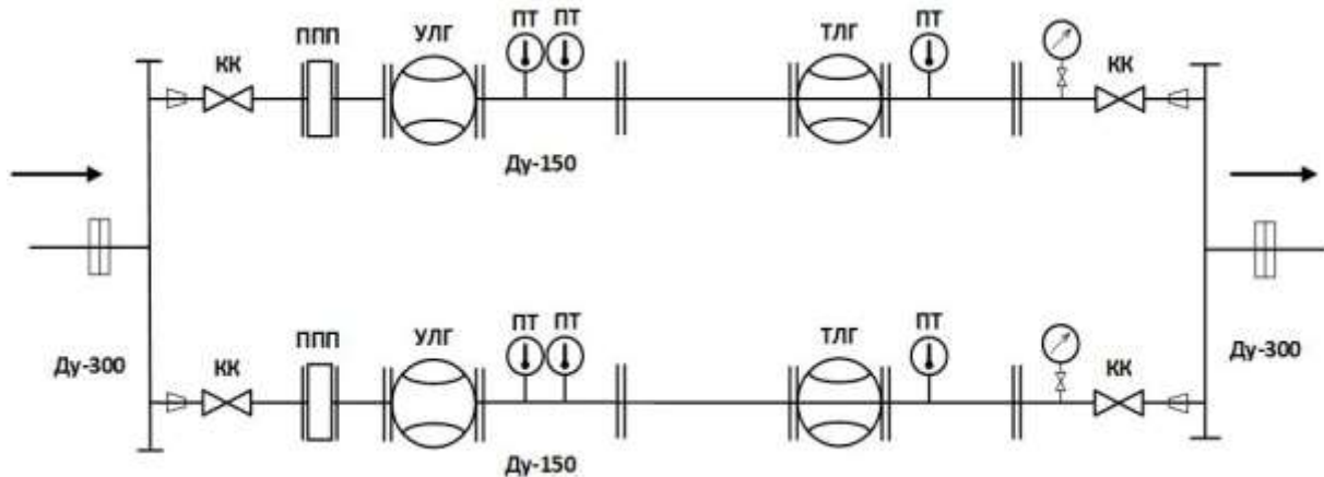
Рисунок 1 –Схема УУГ DN300 PN 6,3 МПа УУГ-Б-2-300-6,3-2УЗ/150-2Т/150
