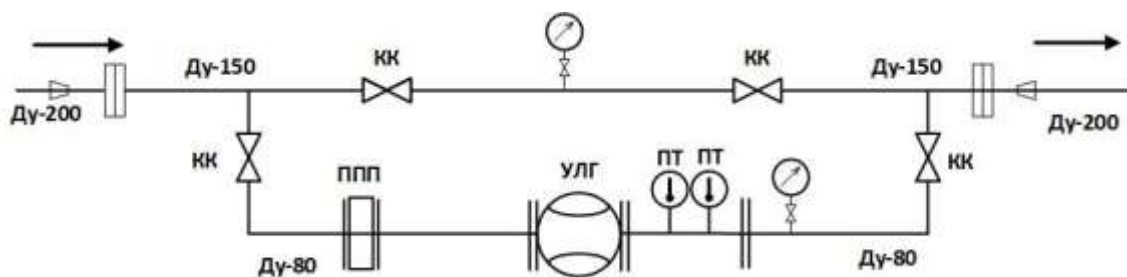
Рисунок 1 –Схема УУГ DN200 PN 6,3 МПа УУГ-Б-1-200-6,3-1УЗ/80
