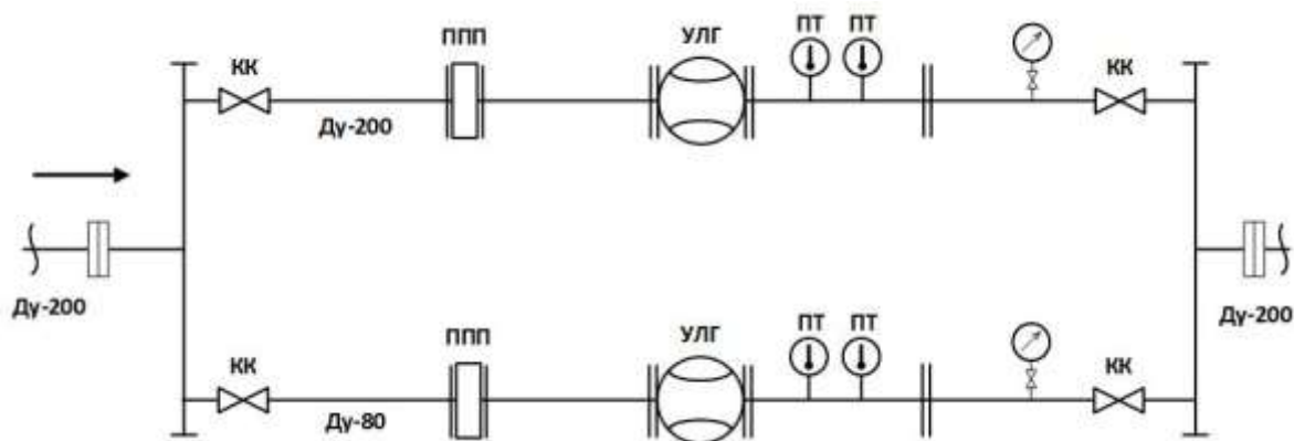
Рисунок 1 –Схема УУГ DN200 PN 1,2 МПа УУГ-Б-2-200-1,2-1УЗ/200-1УЗ/80
