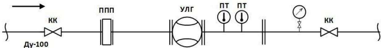
Рисунок 1 –Схема УУГ DN100 PN 6,3 МПа УУГ-Б-1-100-6,3-1/100
